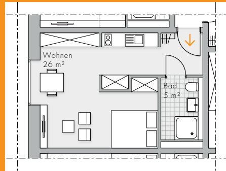
Wohnmodul: MOSAIK architekten bda Nettowohnfläche: 31 m²
